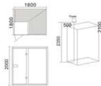
KB-1039 铁杉木 1800x1800x2000mm 可非标订做
