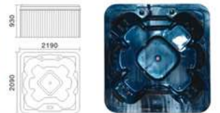
KB-215 2190x2090x930mm
