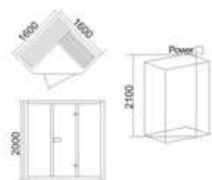
KB-1034 铁杉木 1600x1600x2000mm 可非标订做
